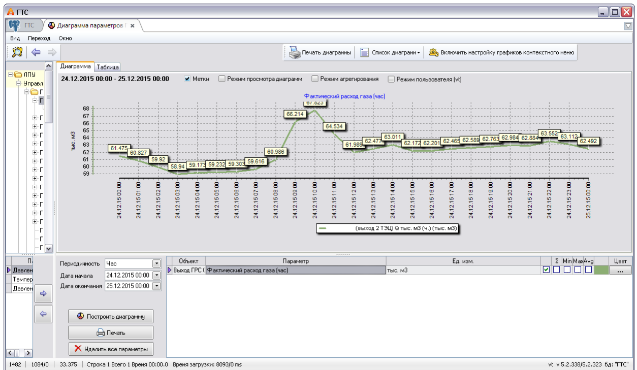
Рис. 5-8 Пример настроенной диаграммы фактического расхода газа
