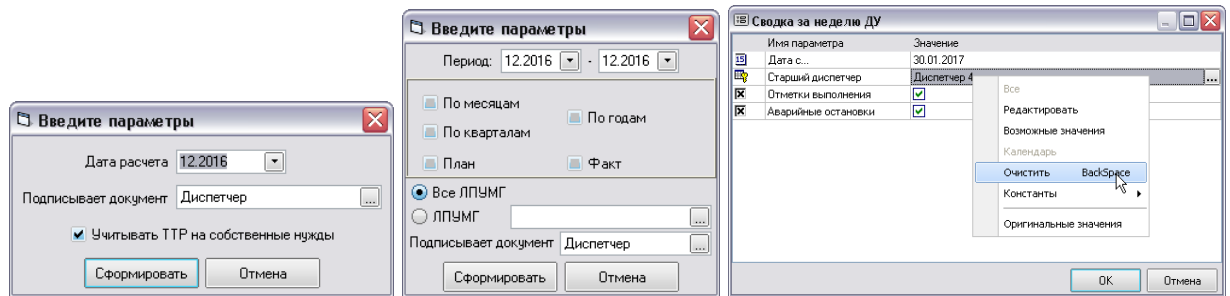
Рис. 12-1 Примеры окон задания параметров отчета
